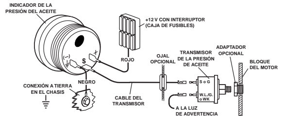
Figura 4. Conexiones del indicador eléctrico de presión de aceite
