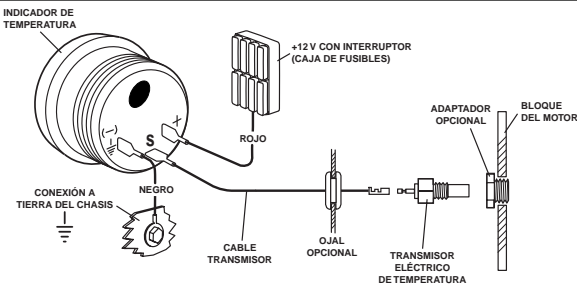
Figura 6. Conexiones del indicador eléctrico de temperatura de agua
