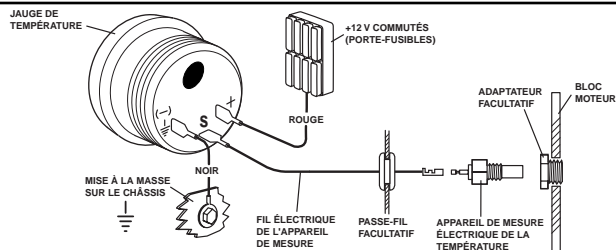
Figure 5. Raccordements de la jauge de température du liquide de refroidissement
