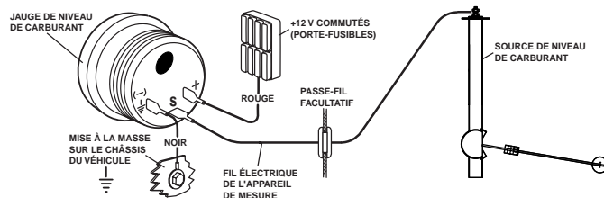
Figure 6. Raccordements de la jauge de niveau de carburant
