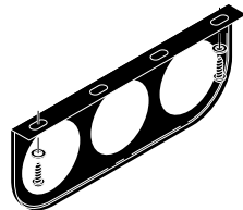
Figura 1. Panel de indicadores
